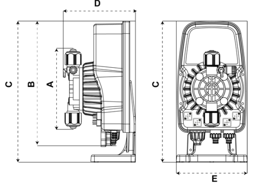
Şekil 2 70'lık Kafa takımı Pompa Ebadı
