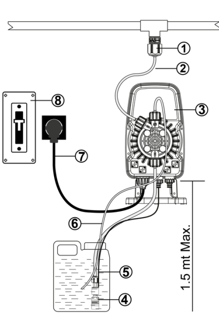
Şekil 10 Cihazın Otomatik hava alma kafalı genel Kurulumu
