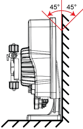
řekil 5 Pompa Dođru Montaj Pozisyonu
